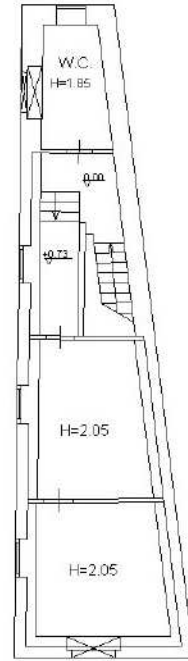
PIANO SECONDO - VILLA
