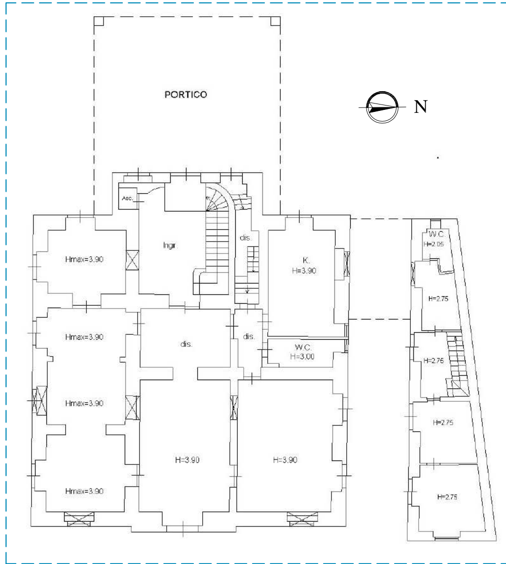
PIANO PRIMO RIALZATO - VILLA
