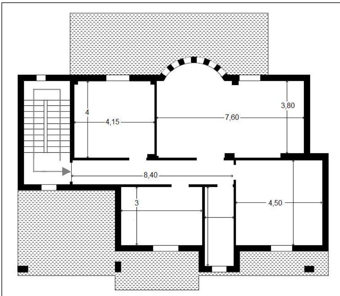
Tavola 5- planimetria del sub 10 (mansarda allo stato rustico al 3° piano)
