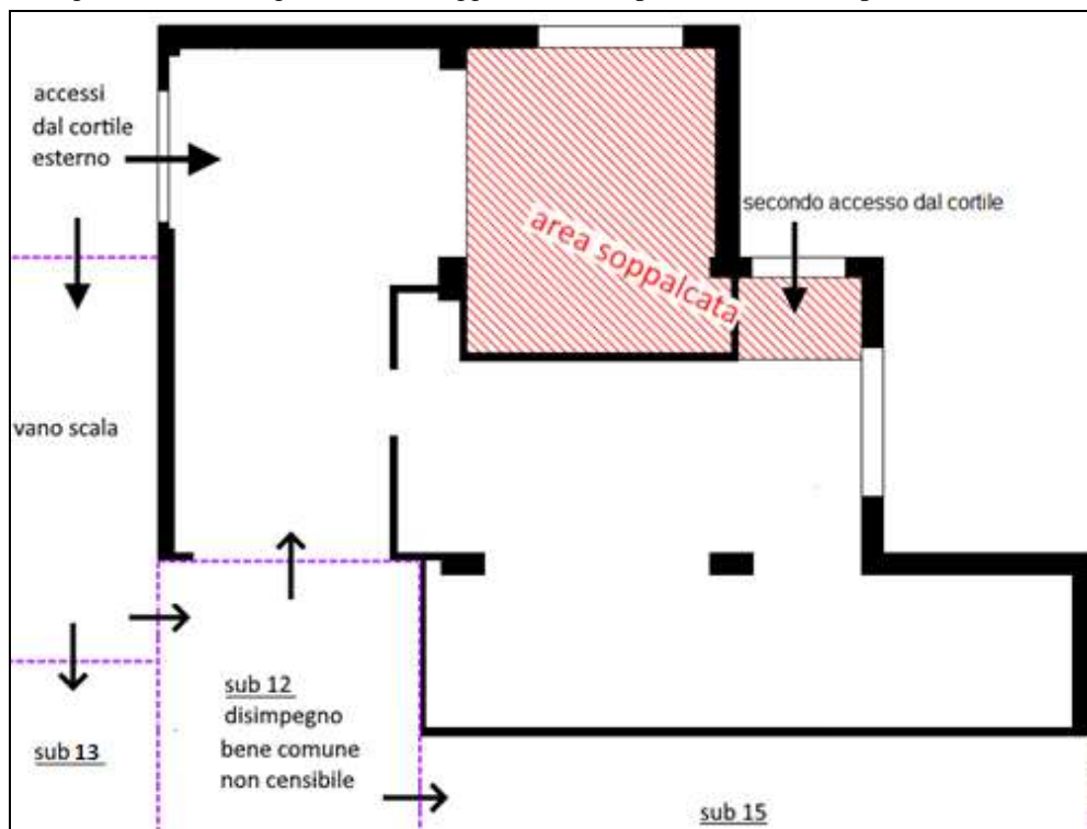
Tavola 8- planimetria del sub 14 (piano seminterrato)
