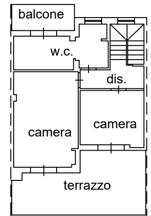
Piano Primo H 2,70 Stato di Fatto - Conforme Planim. Catasto
