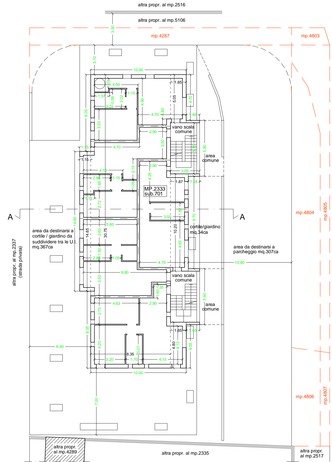
PIANTA p.TERRA
